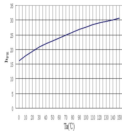
h_{FE} - T_a
