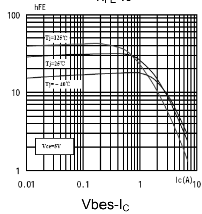
h_{FE}-I_c
