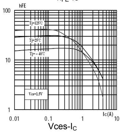
h_{FE}-I_c
