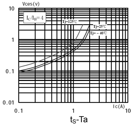
V_{CES}-I_C
