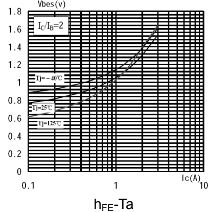
V_{BES}-I_C
