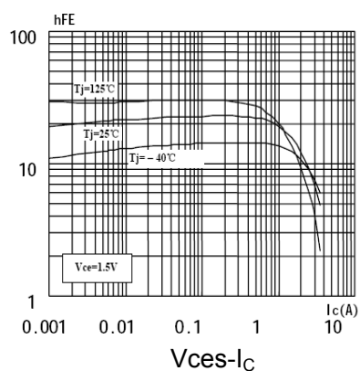
h_{FE}-I_C
