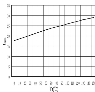
h_{FE}-T_a
