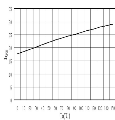
h_{FE}-T_a
