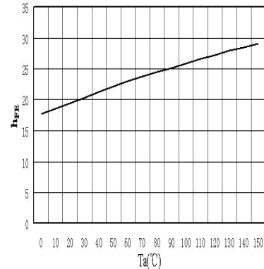
h_{FE}-T_a
