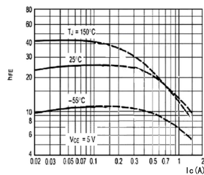
h_{FE}-I_C
