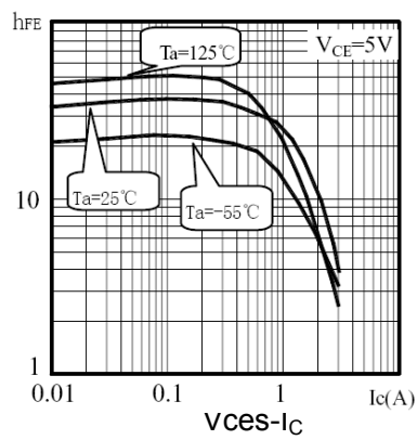
h_{FE}-I_C
