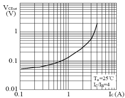
V_{CES} - I_C
