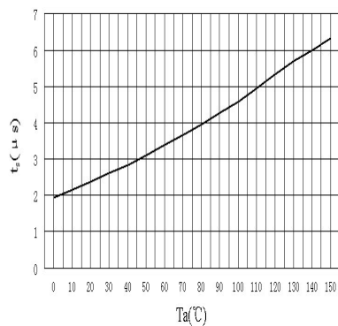
t_s - T_a
