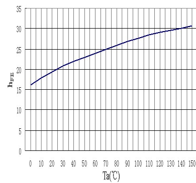
h_{FE} - T_a
