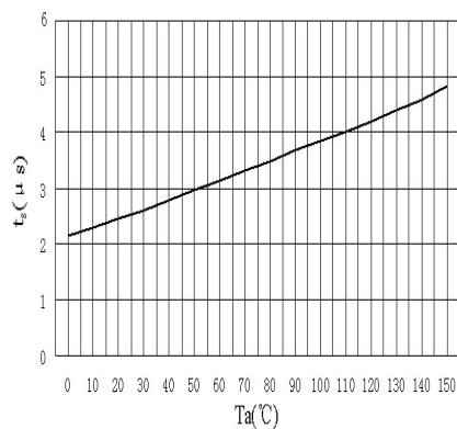
t_s-T_a
