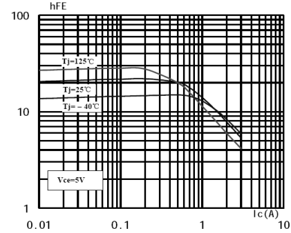
h_{FE}-I_C
