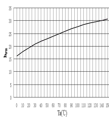
h_{FE} - T_a
