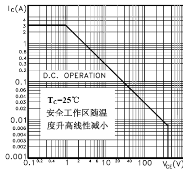
SOA(DC)
