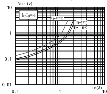
V_{CES}-I_C
