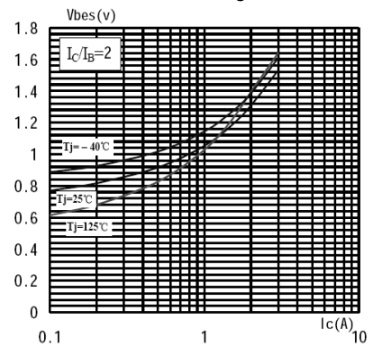
V_{BES}-I_C
