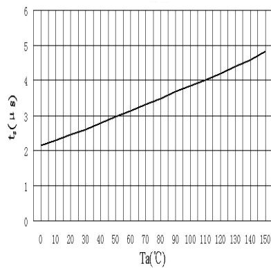
t_s-T_a
