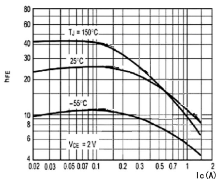
h_{FE} - I_C
