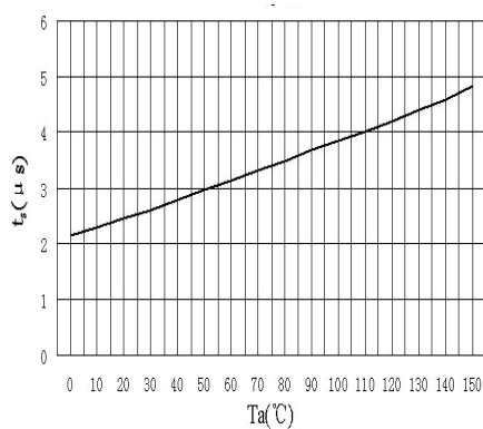
t_s - T_a
