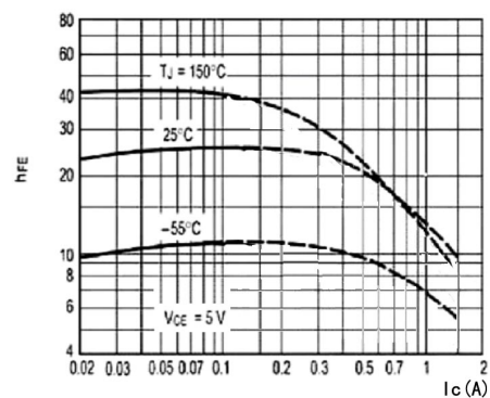
h_{FE} - I_C
