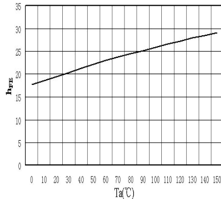
h_{FE} - T_a
