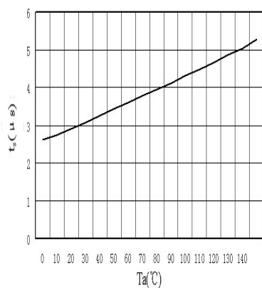
t_s-T_a
