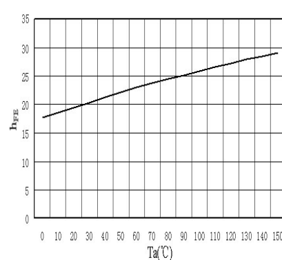
h_{FE}-T_a
