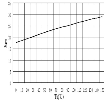
h_{FE} - T_a
