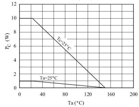
P_C-P_a
