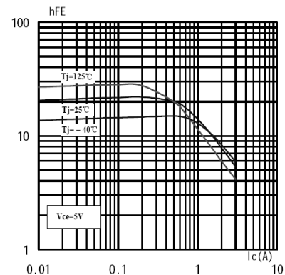
h_{FE}-I_C
