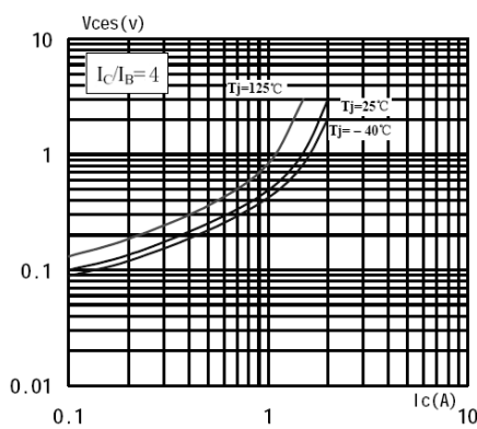
V_{ces}-I_C
