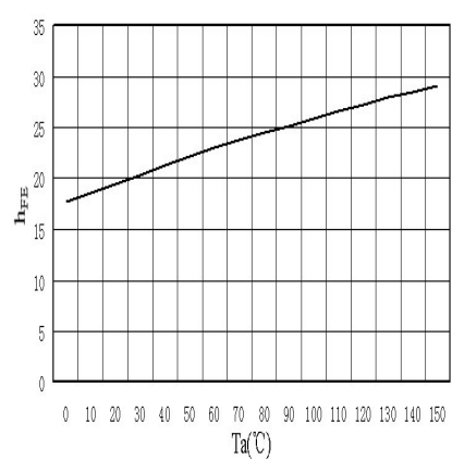
h_{FE}-T_a
