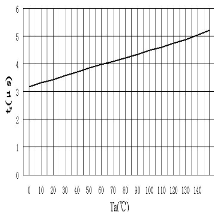
t_s-T_a
