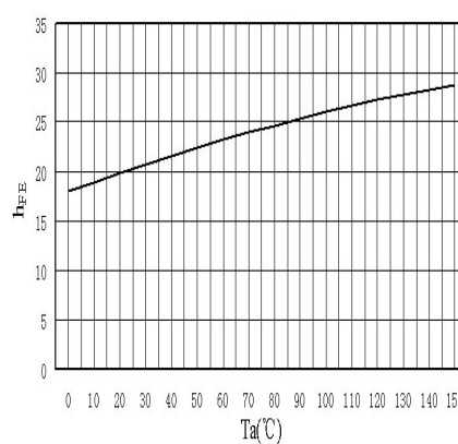
h_{FE}-T_a
