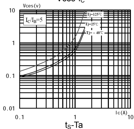
V_{CES}-I_C
