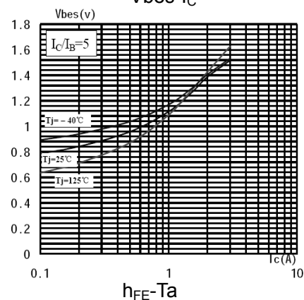
V_{BES}-I_C
